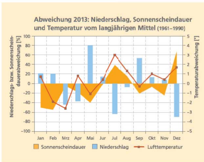
Abbildung 2: Monatliche Abweichungen vom langjährigen Mittel 1961–1990 an den 18 bayerischen Waldklimastationen für das Jahr 2013 für die Größen Niederschlag, Sonnenscheindauer und Lufttemperatur.
